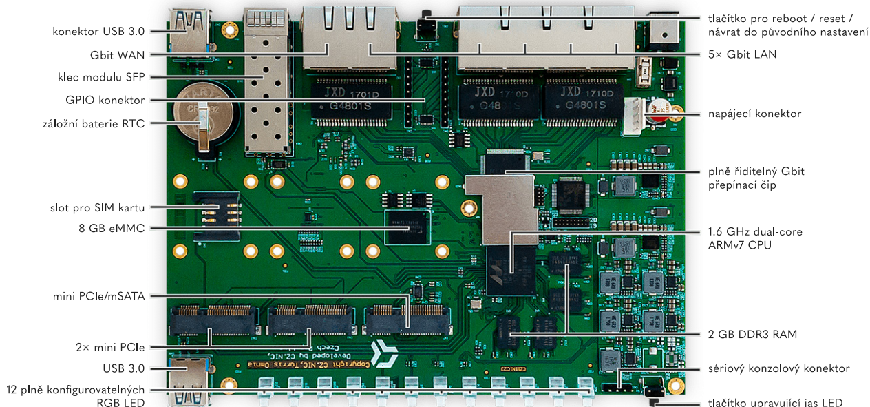
Turrís Omnia No Wi-Fi: komponenty základní desky
